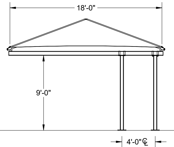
END ELEVATION
